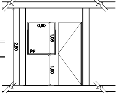
DETALLE TABIQUE CON PAÑO FIJO
